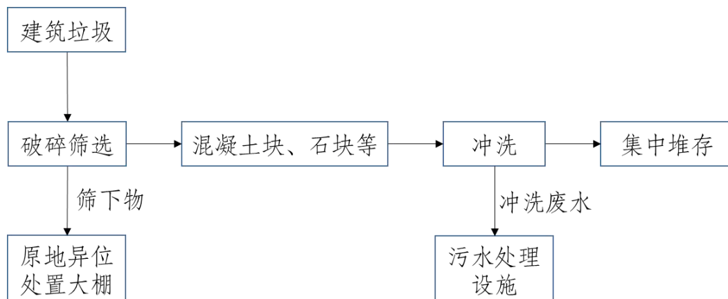
图5-3 建筑垃圾处理流程
