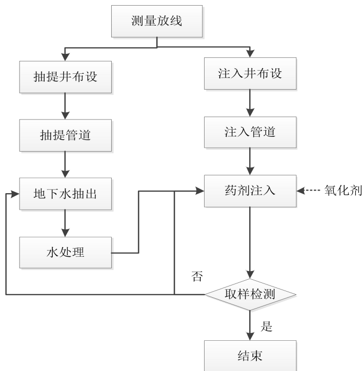
图5-3 地下水处理工艺流程图
